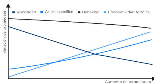
Figura 1.10: Variación de propiedades en función de la temperatura.
