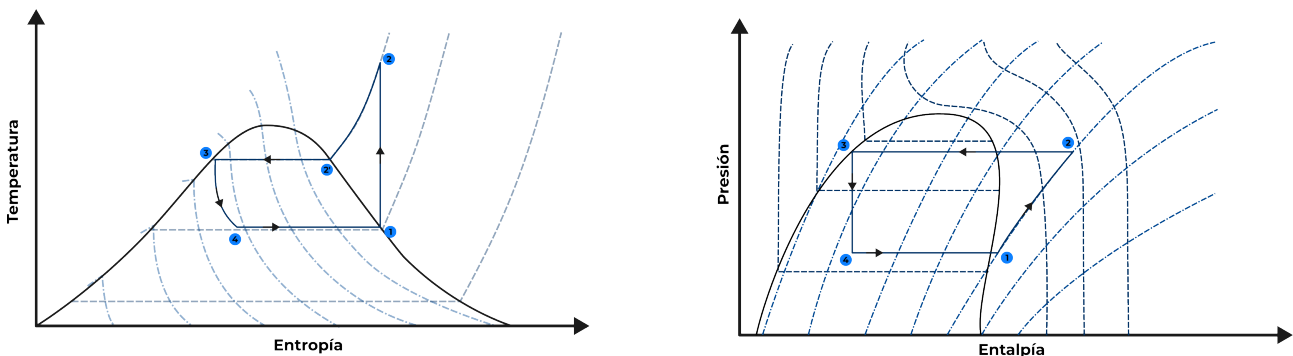
Figura 1.14: Ciclo Rankine inverso.
