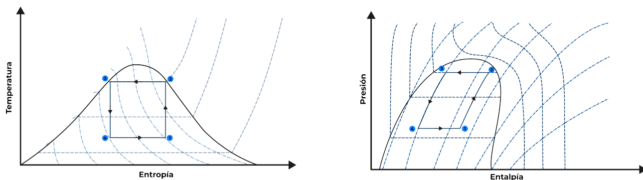
Figura 1.13: Ciclo Carnot Inverso.
