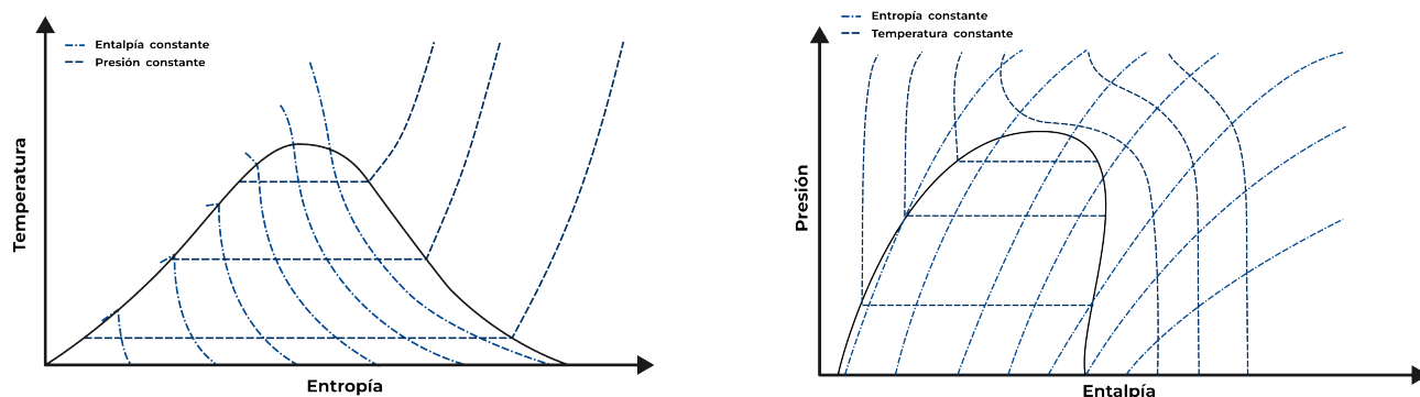
Figura 1.12: Diagramas de T-s y p-h y sus curvas de propiedades constantes.
