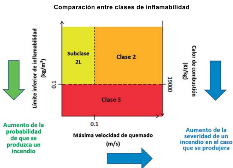
Figura 1.11: Comparación entre clases de inflamabilidad.
